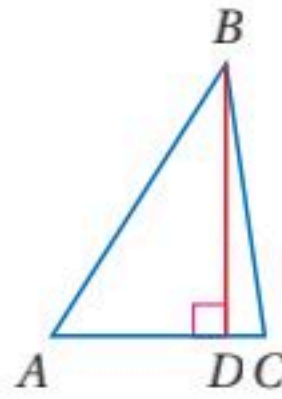
\overline{BD} هو الارتفاع من B إلى \overline{AC} .
