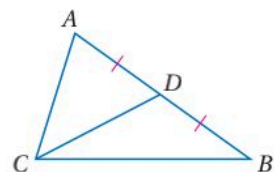
CD قطعة متوسطة في \triangle ABC .
