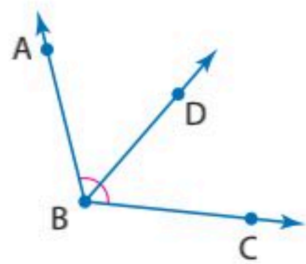
BD منصف لـ \angle ABC
